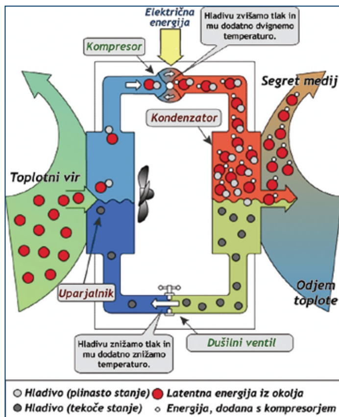
Krožni proces toplotne črpalke
