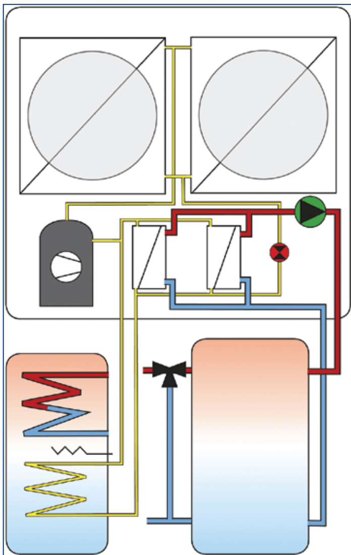
Shema odjema vroče pare za segrevanje sanitarne vode
