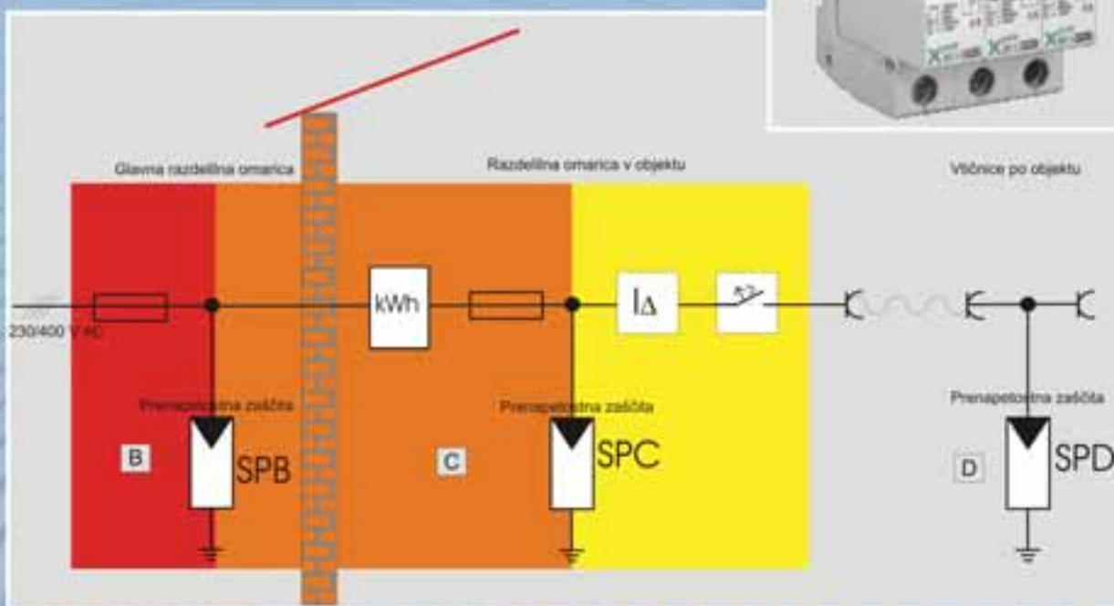
Prikaz delovanja prenapetostne zaščite
